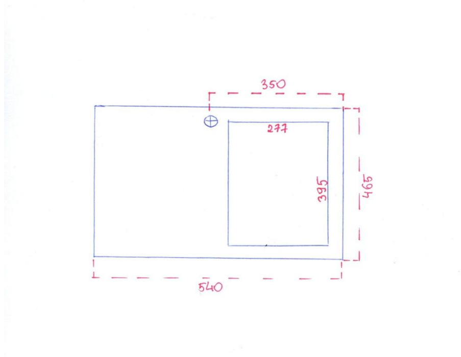
Rys. zlewu z wymiarami
