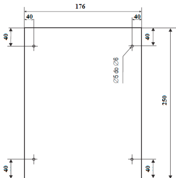
Rys. 3. Fascykula archiwalna B5 176 mm x 250 mm
