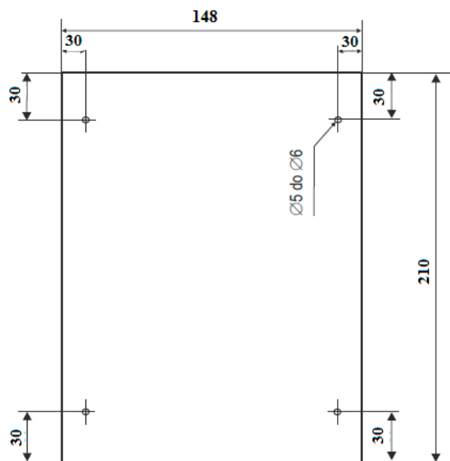
Rys. 2. Fascykula archiwalna A5 148 mm x 210 mm
